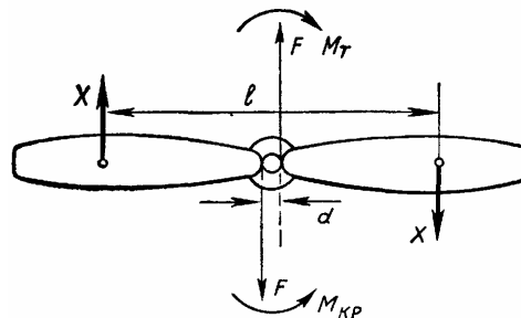
Рис. 69 Тормозящий момент воздушного винта и крутящий момент двигателя
