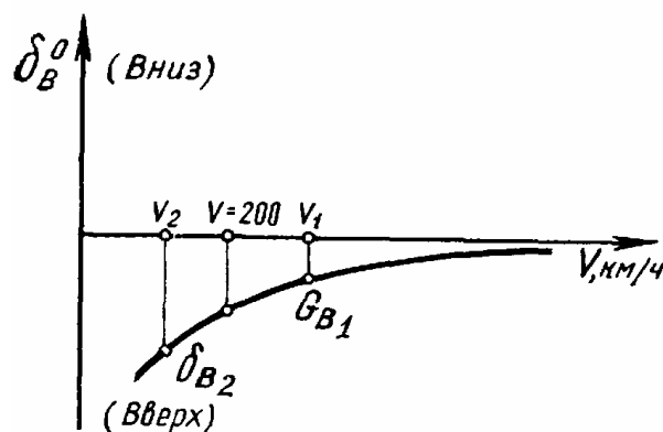
Рис. 137 К объяснению продольной статической устойчивости самолетов по скорости при зафиксированном управлении
