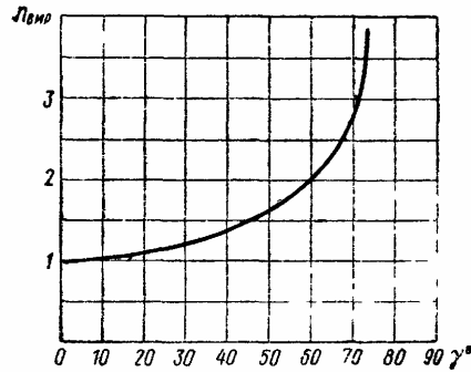
Рис. 179 Зависимость перегрузки на вираже от крена
