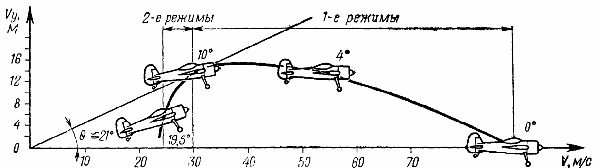
Рис. 90 1-е и 2-е режимы подъема
