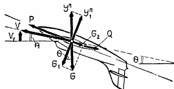
Рис. 207 Схема сил при подъеме в перевернутом полете
