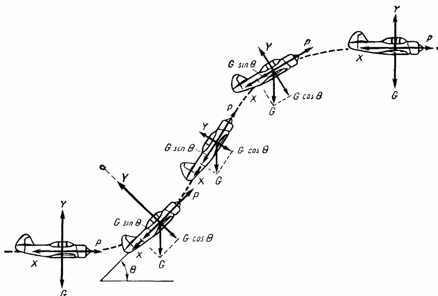
Рис. 189 Схема сил, действующих на самолет на горке
