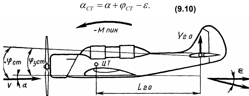
Рис. 132 Момент горизонтального оперения
