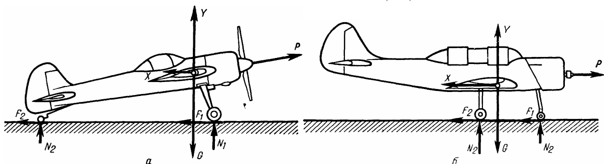
Рис. 112 Схема сил, действующих на самолет Як-55 (а) и самолет Як-52 (б) на взлете
