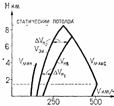
Рис. 87 Изменение характерных скоростей горизонтального полета с подъемом на высоту самолета с поршневой силовой установкой
