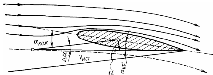
Рис. 35 Отклонение воздушного потока вниз, вызванное вихревым индуктором
