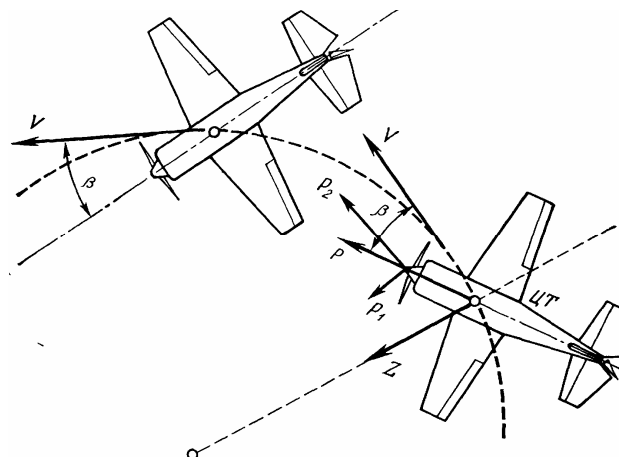
Рис. 185 Плоский вираж с внешним скольжением
