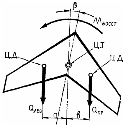
Рис. 154 Влияние стреловидности на путевую устойчивость
