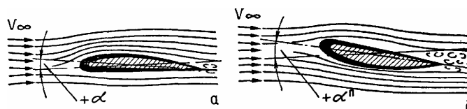
Рис. 199 Картина обтекания профиля крыла в прямом и перевернутом полете
