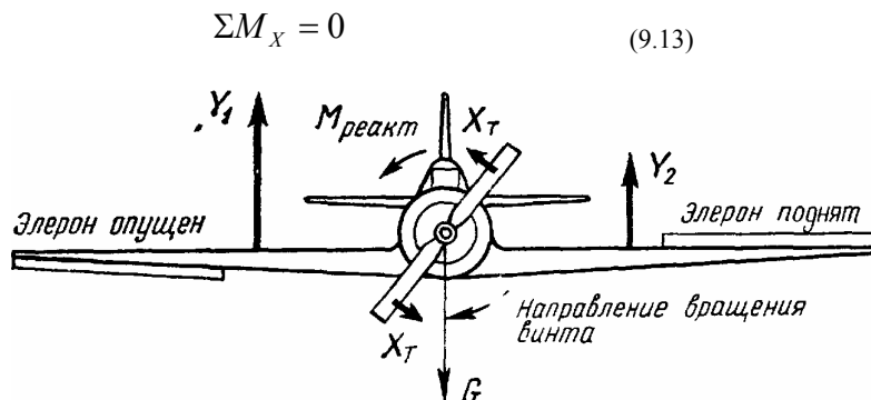
Рис. 139 Реактивный момент воздушного винта и уравнивание его методом отклонения элеронов
