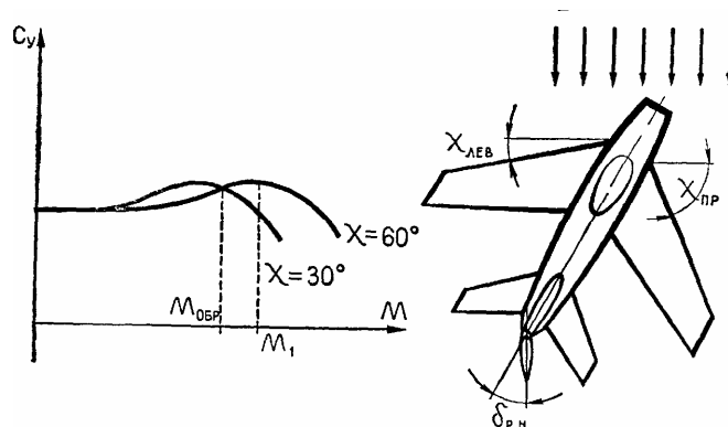
Рис. 149 Изменение C_y в зависимости от числа M полета и стреловидности крыла
