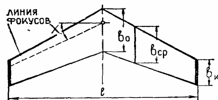
Рис. 24 Геометрические характеристики крыла
