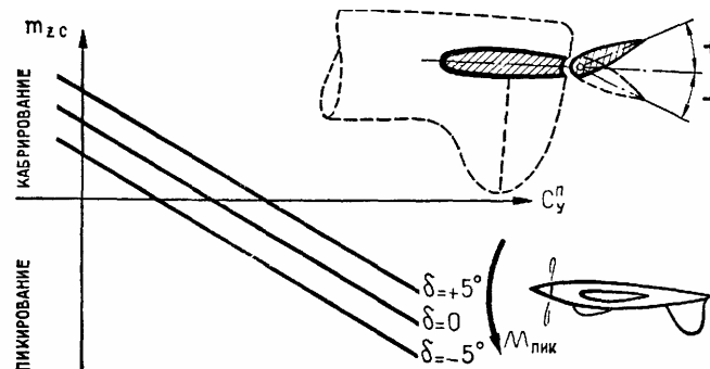
Рис. 204 График m_z = f(C_y^П, \delta) для перевернутого полета
