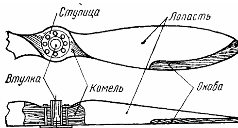
Рис. 60 Воздушный двухлопастный винт неизменяемого шага
