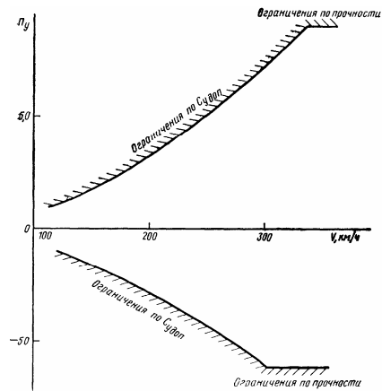
Рис. 176 Располагаемые перегрузки самолета Як-55 при H=1000 м
