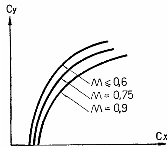
Рис. 46 Поляры самолета для различных чисел M
