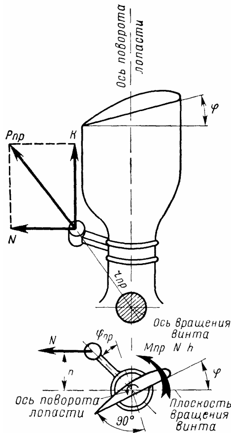
Рис. 74 Характер действия на лопасть воздушного винта собственных центробежных сил
