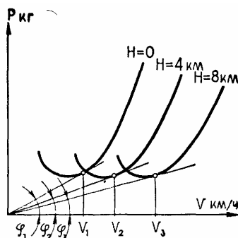
Рис. 218 Зависимость отношения P_n/v от высоты и скорости полета
