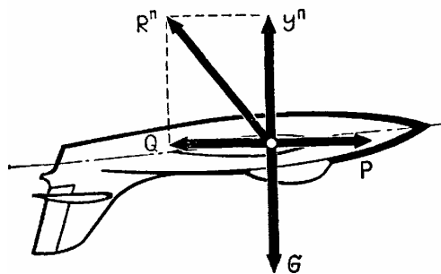
Рис. 206 Схема сил в горизонтальном перевернутом полете
