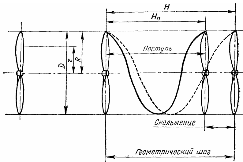
Рис. 63 Диаметр, радиус, геометрический шаг воздушного винта
