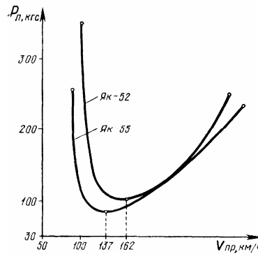
Рис. 81 Кривые потребных тяг для горизонтального полета самолетов Як-52 и Як-55
