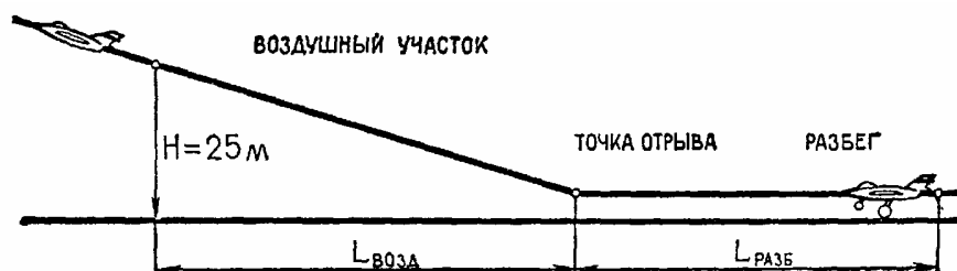
Рис. 105 Схема взлета самолета
