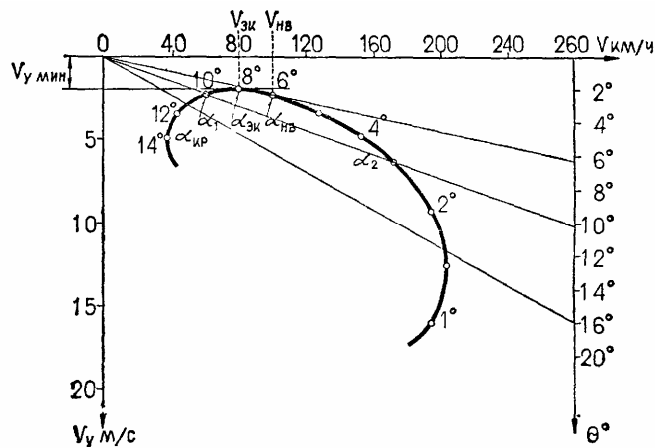
Рис. 98 Поляра скоростей планирования
