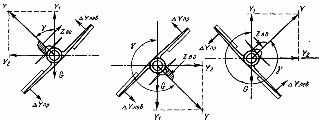
Рис. 193 Схема сил, действующих на самолет при выполнении горизонтальной штопорной бочки
