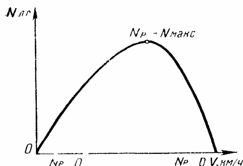
Рис. 71 Примерный вид кривой изменения располагаемой мощности в зависимости от скорости полета
