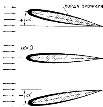
Рис. 27 Углы атаки крыла
