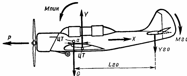
Рис. 126 Условия продольного равновесия самолета в горизонтальном полете
