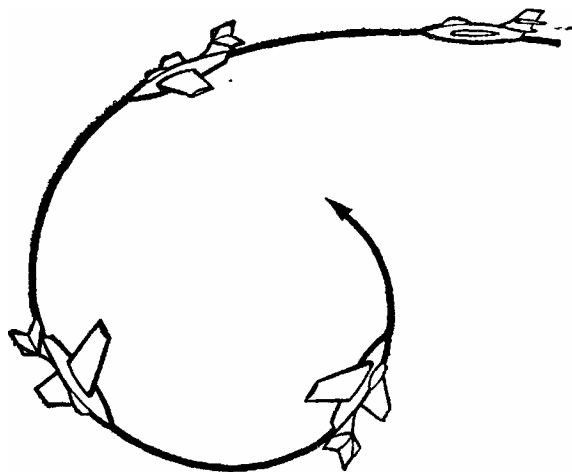
Рис. 157. Спиральная неустойчивость самолета
