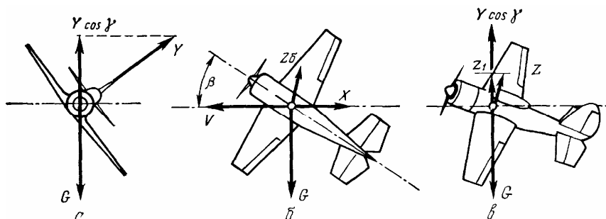
Рис. 184 Глубокий левый вираж с внутренним скольжением
