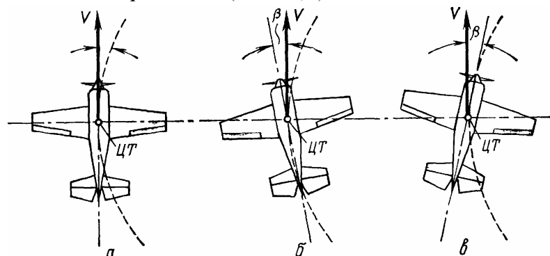
Рис. 177 Схемы виражей: а - правильный виращ; б - виращ с внутренним скольжением; в - виращ с внешним скольжением
