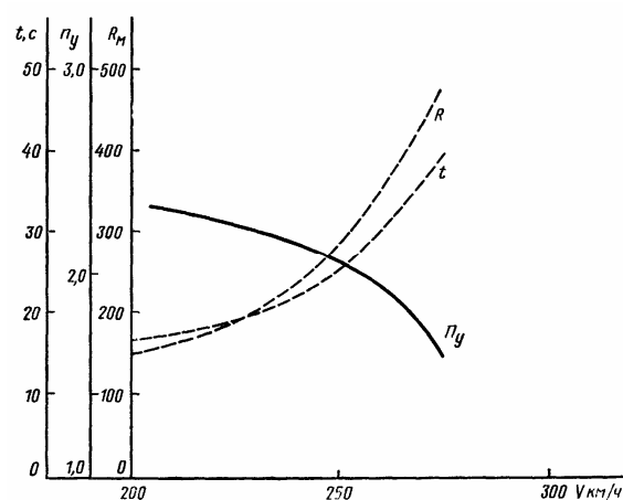
Рис. 182 Характеристики виража самолета Як-52 ( H=1000 м, G_{вз}=1290 кгс, режим работы двигателя-1-й номинал)
