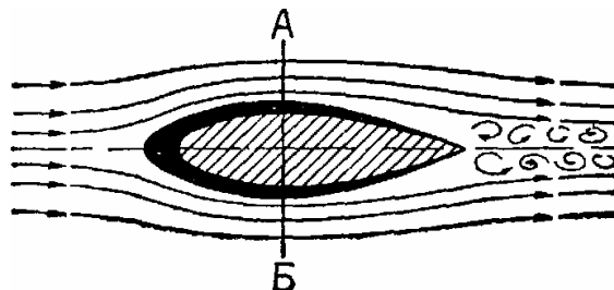
Рис. 18 Аэродинамический спектр удобообтекаемого тела
