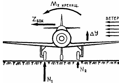
Рис. 108 Взлет самолета с боковым ветром
