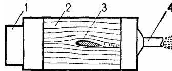
Рис. 16 Дымканал
