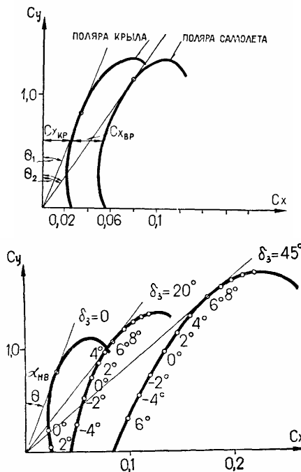
Рис. 44 Поляры крыла и самолета
