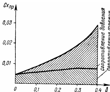
Рис. 33 График зависимости профильного сопротивления от толщины профиля
